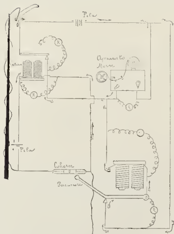
Circuito ricevente.
